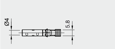
作为单独零件的触子
