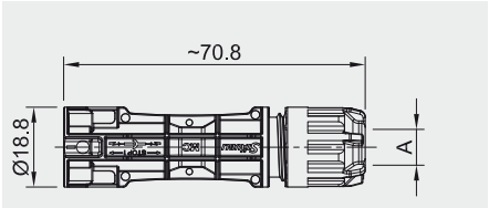
插头 PV-KST4-EVO 1/6X
