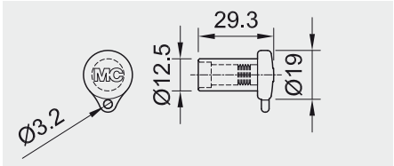
插座保护帽(PV-BVK4)
