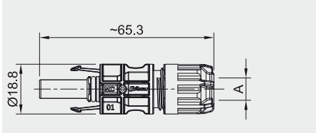
插座 PV-KBT4-EVO 1/6X
