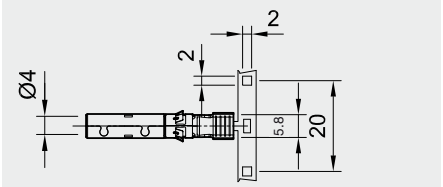
卷盘上的触子
